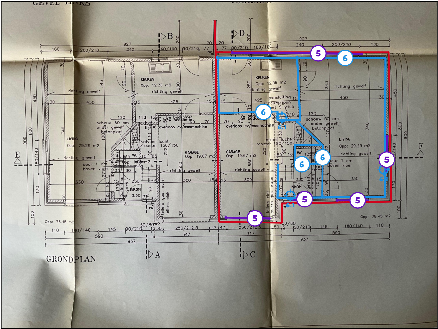
Legende van plan 1.1: Gelijkvloers
