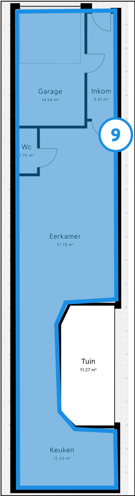
Legende van plan 1.12: Verdiep 0 aanduiding plafonds
